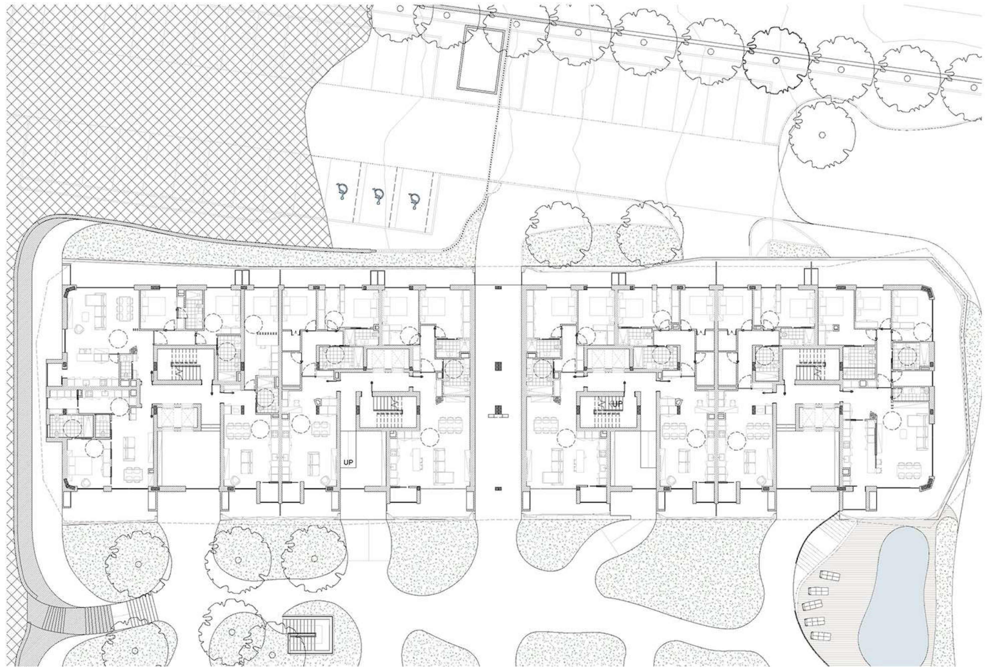
PISO RC | ESCALA: 1 : 200
