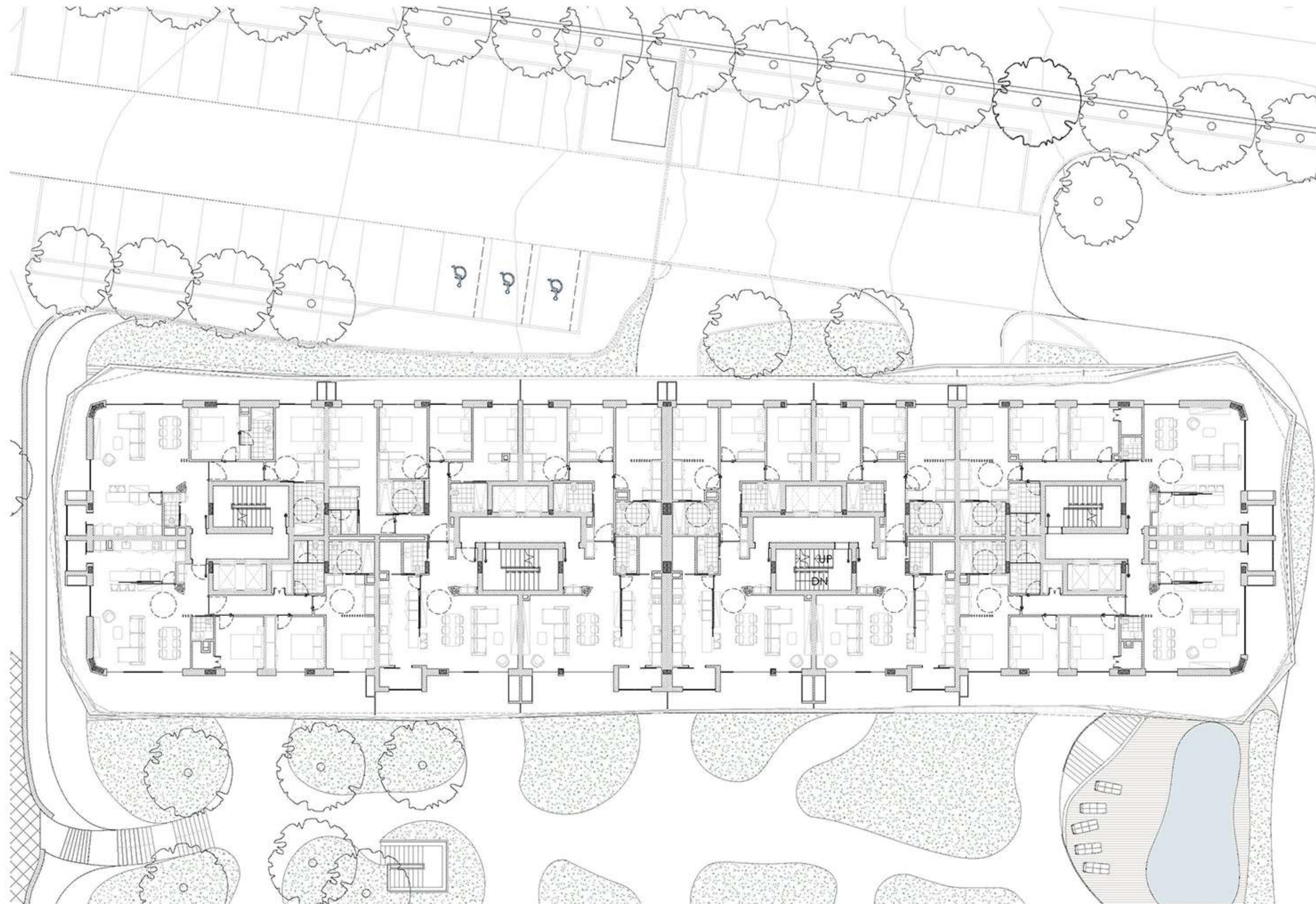
PISO TIPO | ESCALA: 1 : 200
